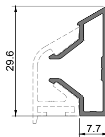
SA 31 Perfil complementar Complementary profile Profilé complémentaire
