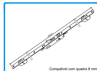
201207 FECHADURA PINOS TESTA INOX T25 U C/1600
