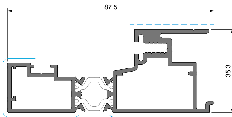
FC 48 Perfil de remate Finishing profile | Profilé de finitions
