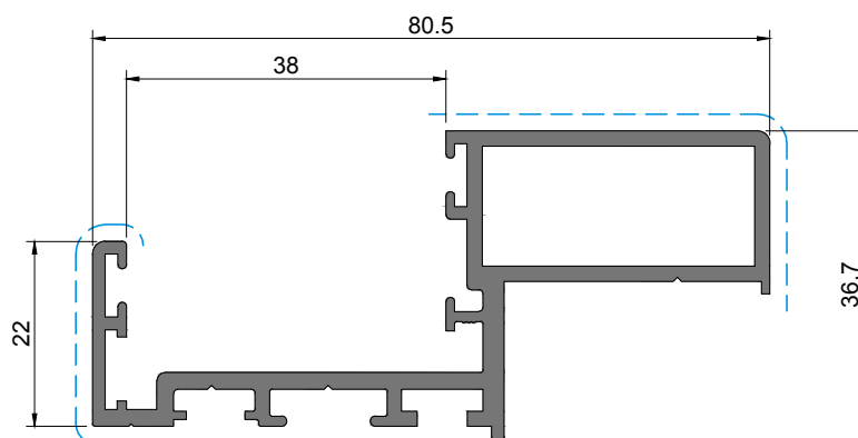
FC 60 Perfil para quadros Frames profile | profilé pour cadres
