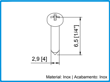
290060 PARAF. DIN7981 PH 2,9x6,5 INOX A2
