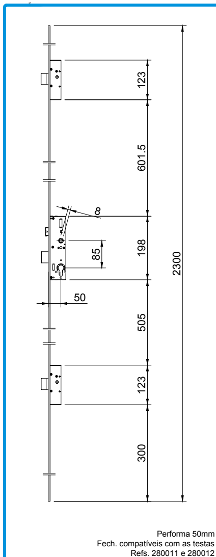
201082 FECH. 3 PONTOS PERFORMA 50mm
