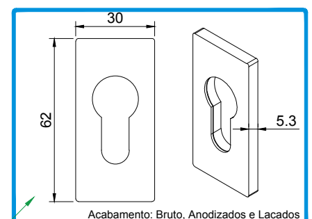
220197 ESPELHO ALUMÍNIO 30MM P/
