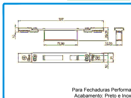
280011 TESTA SUP/INF 22x197 PARA
