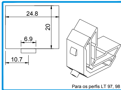
204020 ESQUADRO LT 24,8 x 20-D
