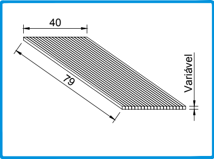
218113 CALÇO PARA VIDRO 79x40x2
