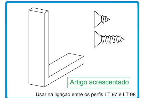
204021 ESQ. ALINHAMENTO LT97/LT98
