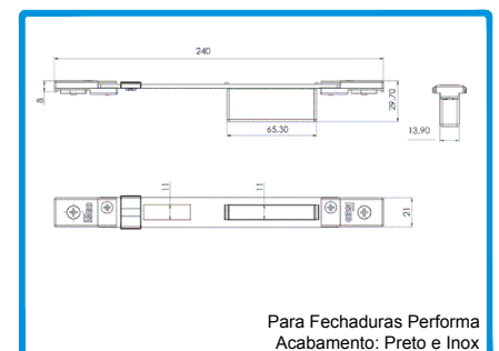
280012 TESTA CENTRAL 22x240 PARA
