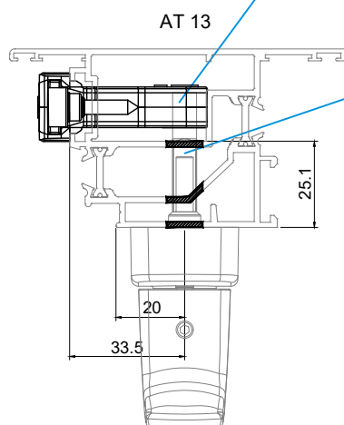
203018 CAIXA TRANSM. BIDIRECIONAL 33,5MM
