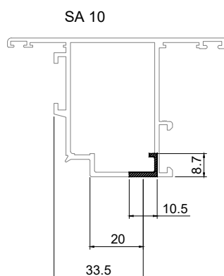
203018 CAIXA TRANSM. BIDIRECIONAL 33,5MM
