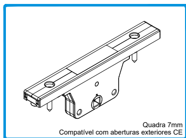
203018 CAIXA TRANSM. BIDIRECIONAL 33,5MM
