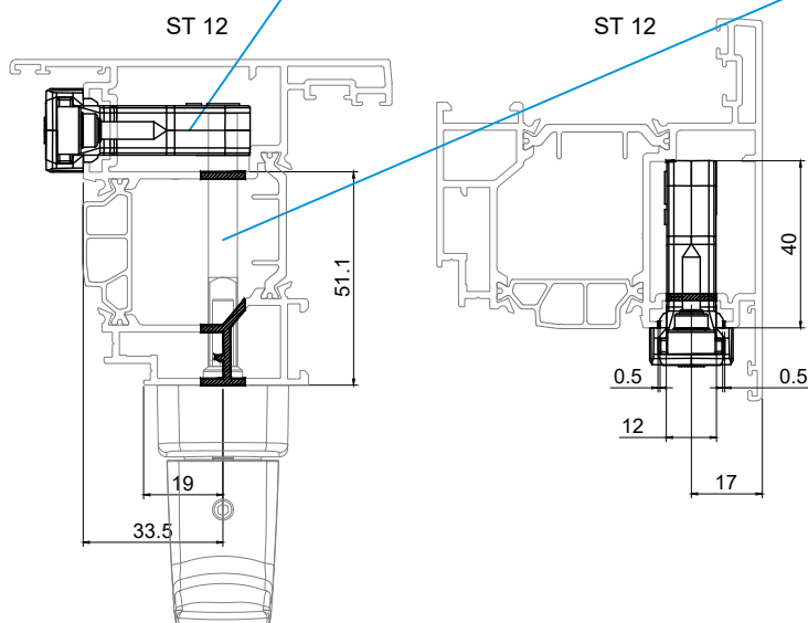
203018 CAIXA TRANSM. BIDIRECIONAL 33,5MM
