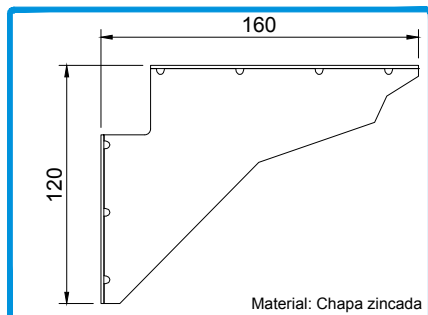
230316 SUPORTE FIXAÇÃO 160MM
