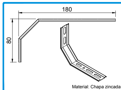
213311 ÂNGULO FIXAÇÃO 180MM
