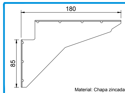
230317 SUPORTE FIXAÇÃO 180MM
