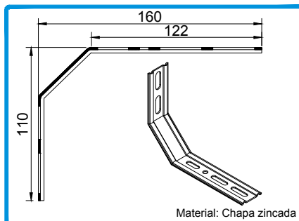
213235 ÂNGULO FIXAÇÃO 160MM
