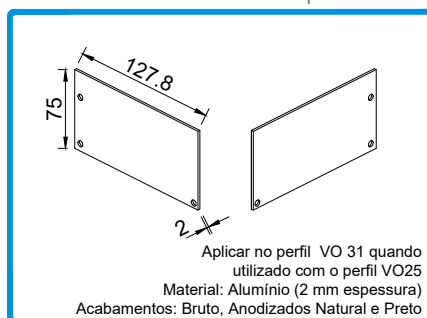
212345 CONJ. TOPOS CALEIRA/SOL ALTA OS-PIVOT
