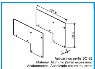
212351 CONJ.TOPOS CALEIRA/SOL BAIXA OS-PIVOT
