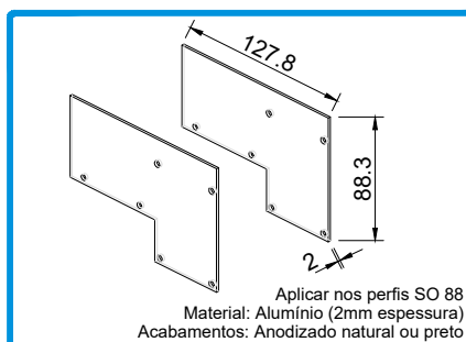
212351 CONJ. TOPOS CALEIRA/SOL BAIXA OS-PIVOT
