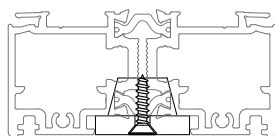
OS 80 Padeira Door lintel | Linteau
