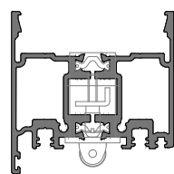
OS 75 Perfil móvel lateral Lateral mobile profile | Cadre ouvrant latéral
