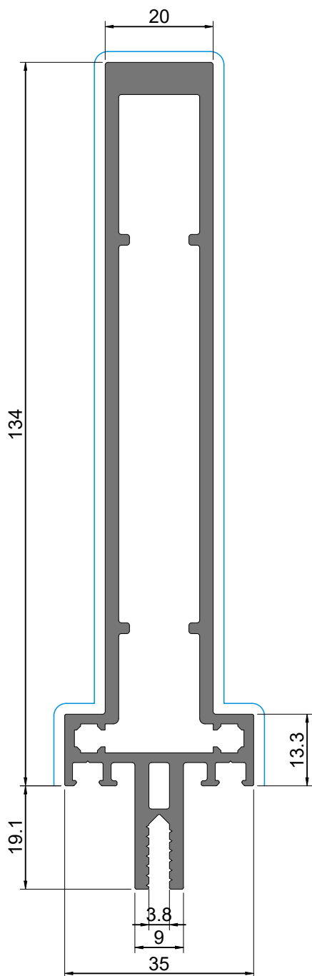
FC 94 Perfil complementar Complementary profile Profilé complémentaire
