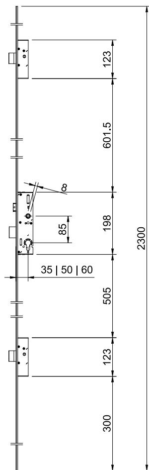
201615 FECH. 3 PONTOS PERFORMA 35mm
