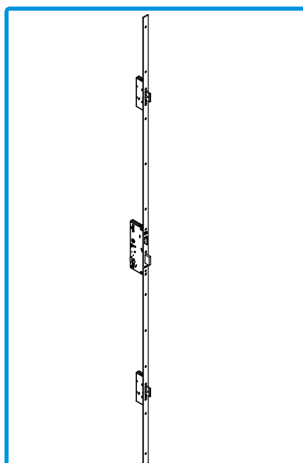
Fechadura 3 pontos para os perfis IT 12/93, LT12/93 e ST 12/93, compatível com testas Ref. 280011 e 280012, 201093 FECHAD. 3 PONTOS PERFORMANCE 60MM
