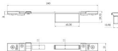
280011 TESTA SUP/INF 22x197 PARA FECHADURA PERFORMA
