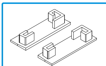
Aplicar nos perfis LT 93, LT 93 e ST 93 Material: ABS | Acabamento: Preto
