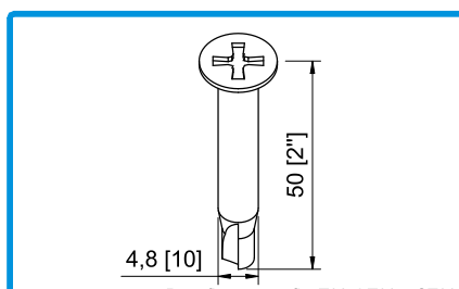
Para fixar os perfis IT93, LT93 e ST93 aos perfis IT12, IT78, LT11, LT 12 e ST11 e ST12 Material: Inox | Acabamento: Inox
