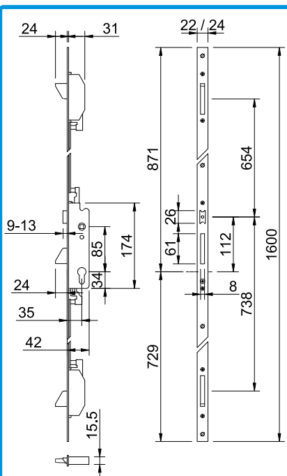
201179 FECHADURA 3 PONTOS 7717x35
